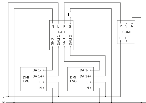
Diagrama electrónico interconexión maestro-maestro
